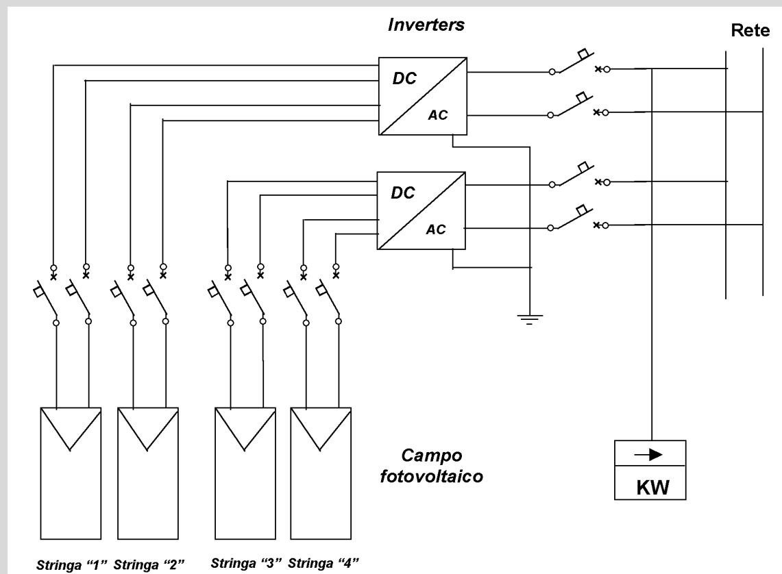
Figura 9 - Schema elettrico indicativo di un impianto fotovoltaico connesso in rete
